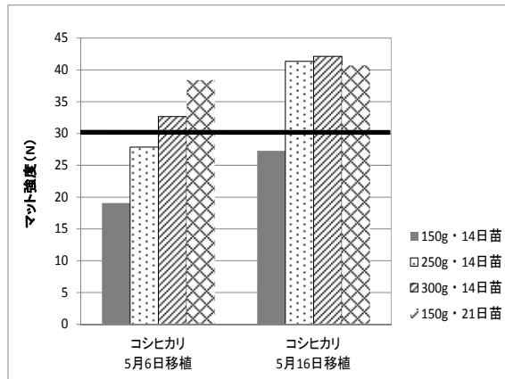
図1 苗のマット強度 (N)
