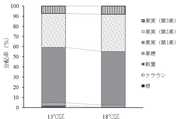
図3 異なる日中の気温が 13 CO 2 施与24時間後の分配率に及ぼす影響
